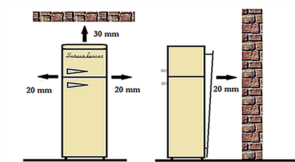
Mindestabstände
