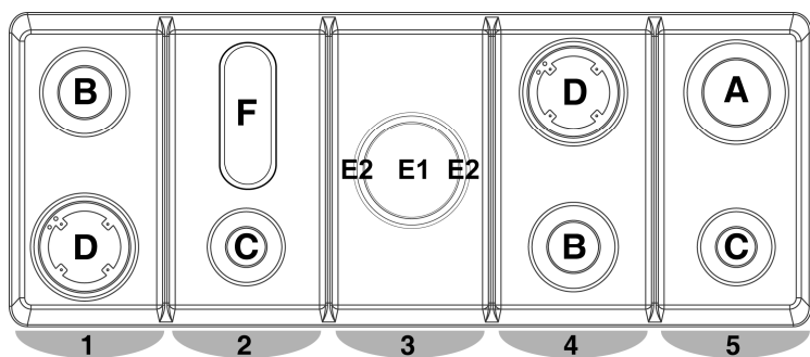
ALGEMENE TABEL VOOR DE SPROEIERS (ALUMINIUM)
